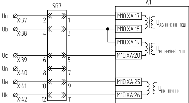
Цепи переменного и напряжения А1
