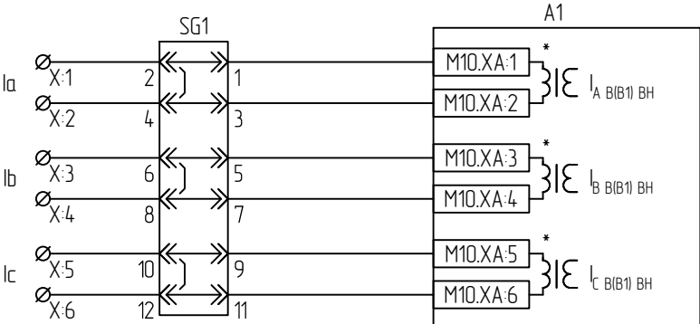
Цепи переменного тока А1
